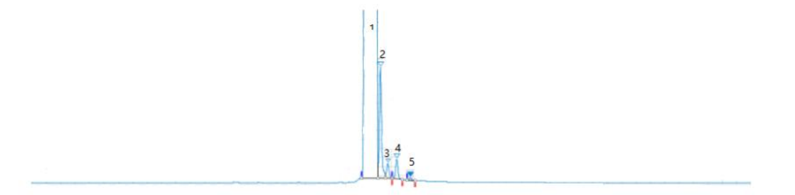
图 1 二甲基二乙烯基硅烷的典型色谱图
