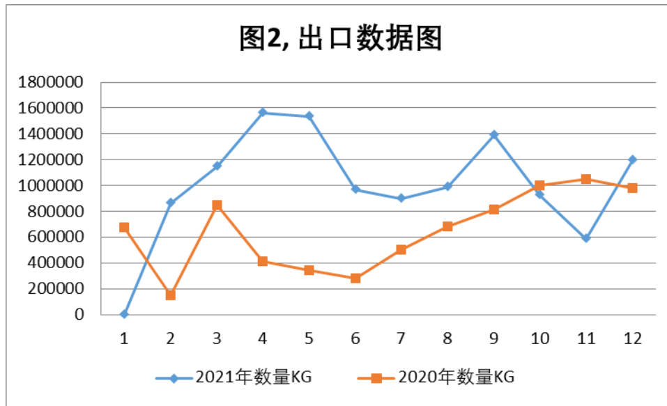
图2 六氟磷酸锂出口数量曲线
