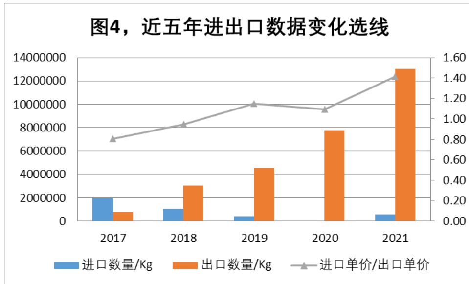
图4 近五年六氟磷酸锂进出口趋势图
